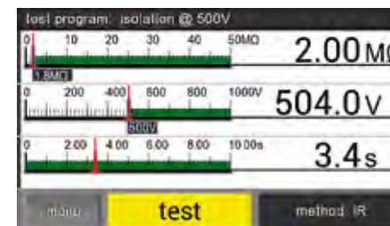
Tester rezystancji izolacji
